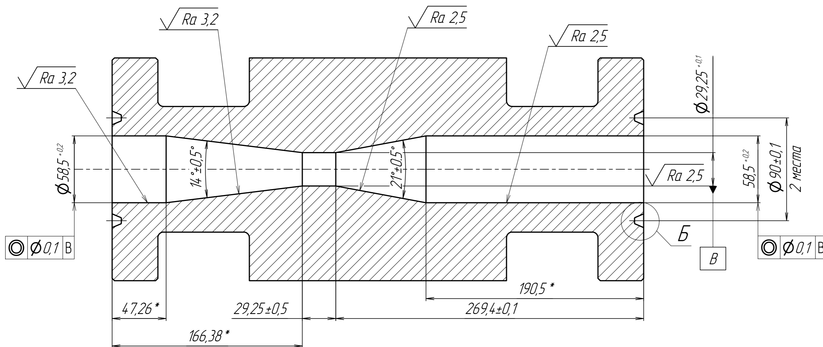
A-A (1:2)
