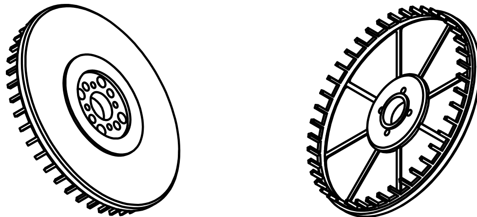
АксонOMETрические виды. M 1:1
