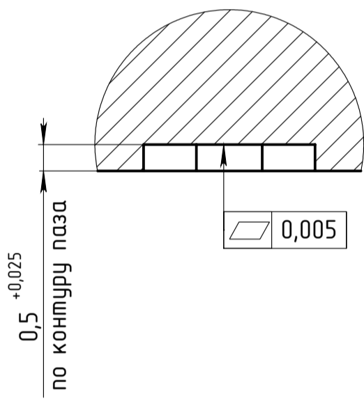
Г (10 : 1)
