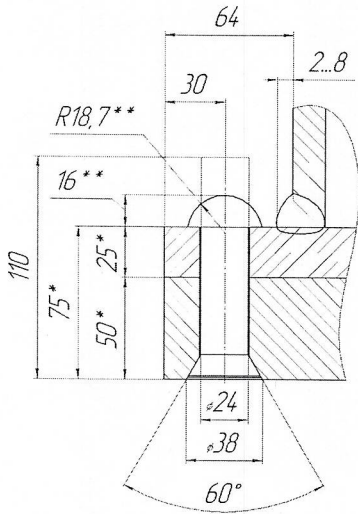
Заклепка 24x110.10 ГОСТ 10300-80
