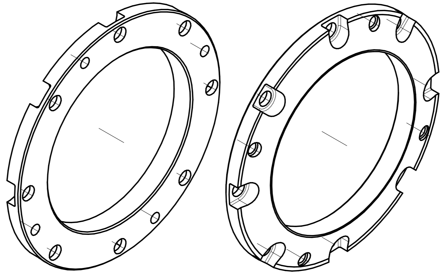
АксонOMETрические проекции (1:2,5)
