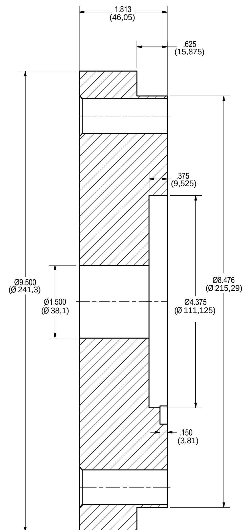
SECTION A-A SCALE 1 : 1
