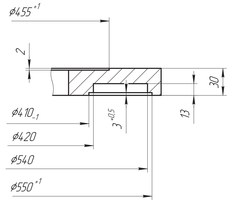
A-A(1:2)
