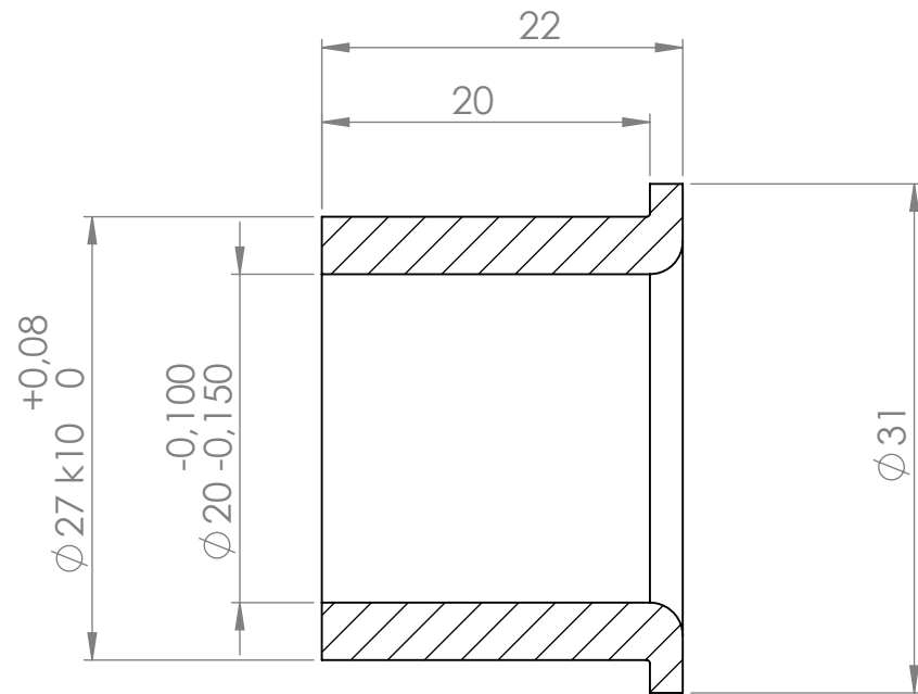
СЕЧЕНИЕ А-А
