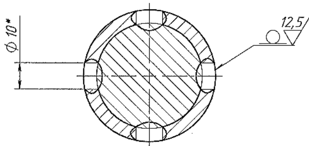
A-A (1:1)
