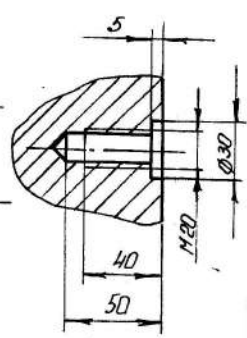
Д-Д M1:2
