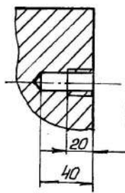
Г-Г M1:2
