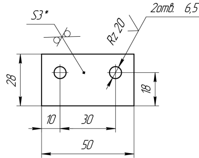
Дет. поз 2
